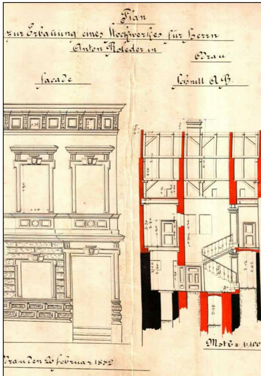
Stavební plán úprav domu čp.28 na Hranické ulici v roce 1882 za majitele oderského městského lékaře Antona Rolledera. Úprava zahrnovala přístavbu 1. patra domu (viz červeně označená část plánu). Návrh pravděpodobně zpracoval oderský stavitel Ludwig Wanke (*1839 / †1897). Muzejní spolek Rolleder, o. p. s.
